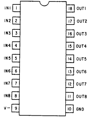
MSL915RS MSL917RS
