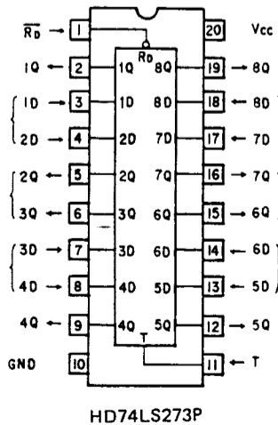
HD74LS273P
