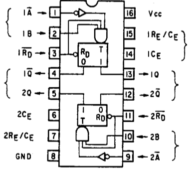
H74LS123P
