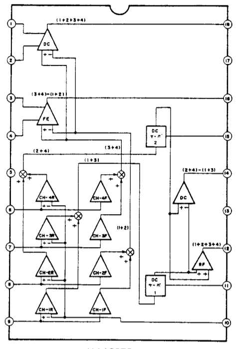
HA12050
