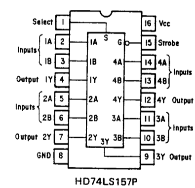
HD74LS157P
