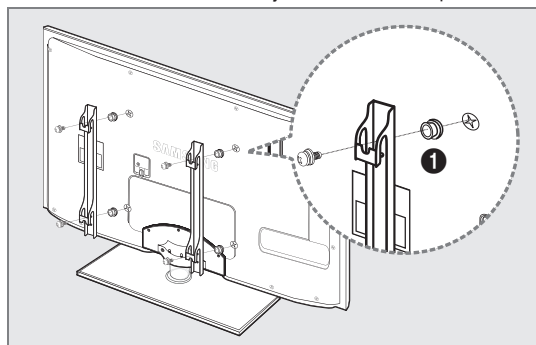
Caso B. Instalación del montaje mural de otra empresa
