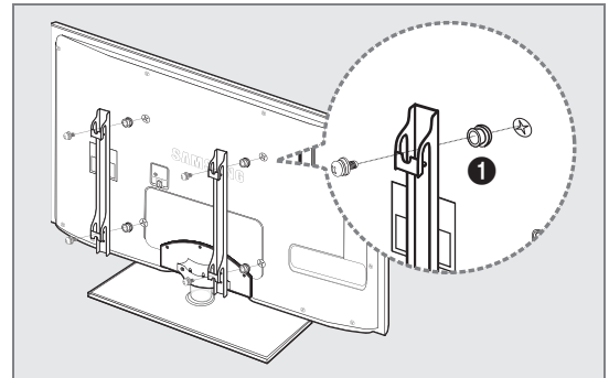
Durum B. Diğer şirketin Duvar Askısının takılması
