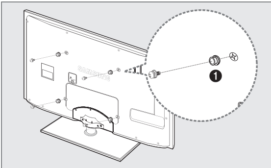
Durum A. SAMSUNG Duvara Montaj Kitinin takılması
